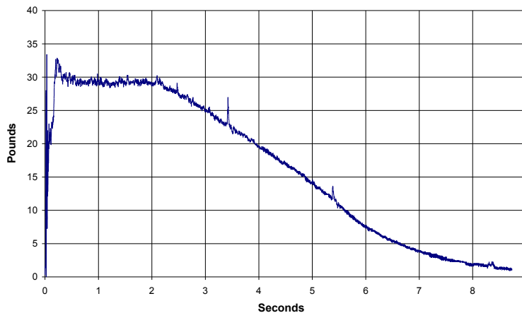
Aerotech I65W DMS
